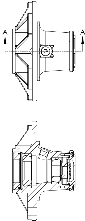
SECTION A-A
